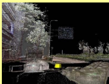
移動計測装置(ペガサス)
