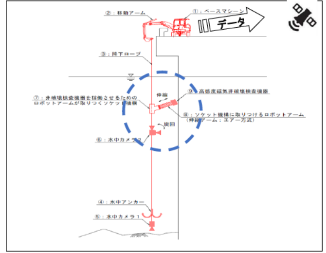
岸壁点検支援ロボット
