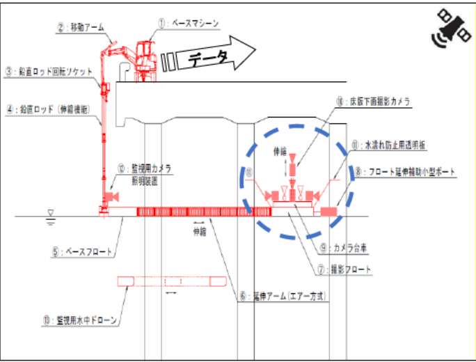
栈橋点検支援ロボット
