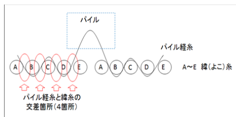
5ピック織り模式図
