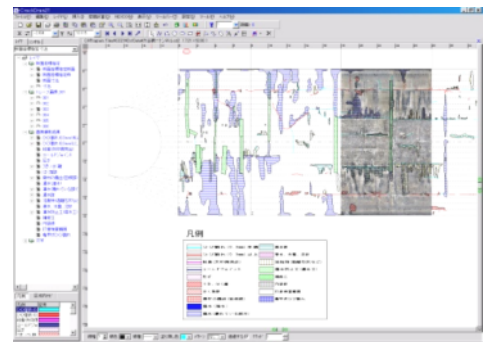
変状展開図作成例
