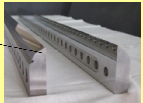
特殊HIP素材への超精密研削加工によるTダイ金型 及び ダイリップ
