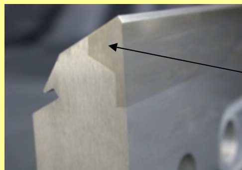
特殊HIP素材への超精密研削加工によるTダイ金型 及び ダイリップ
