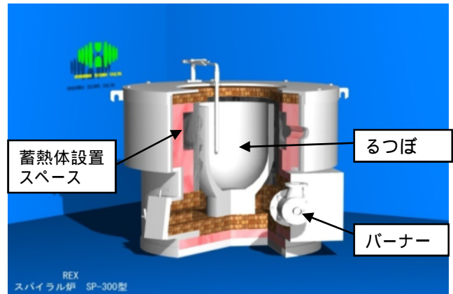
省エネルギー・高効率のアルミ溶解るつぼ炉 断面図
