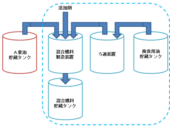
【混合燃料製造システム】
