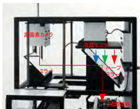
基板画像検査装置内部機構
