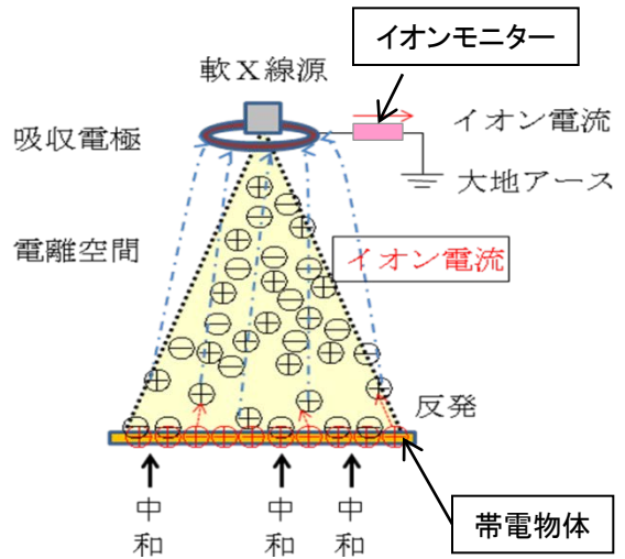
軟X線照射式静電気除電装置の外観と除電原理
