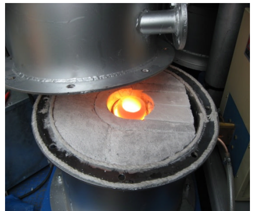
溶融機
