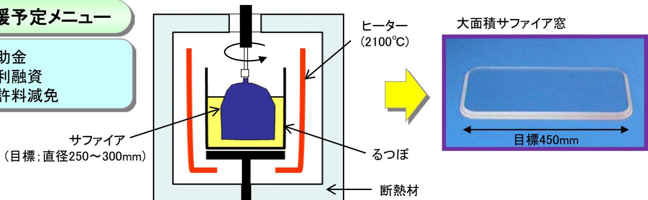
TSMG法(特許技術)による サファイア製造の模式図
