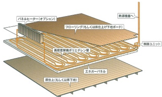
太陽光集熱器を熱源とした給湯及び床暖房システム
