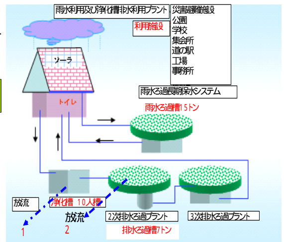
自然式雨・排水ろ過長期保水プラントフロー図
