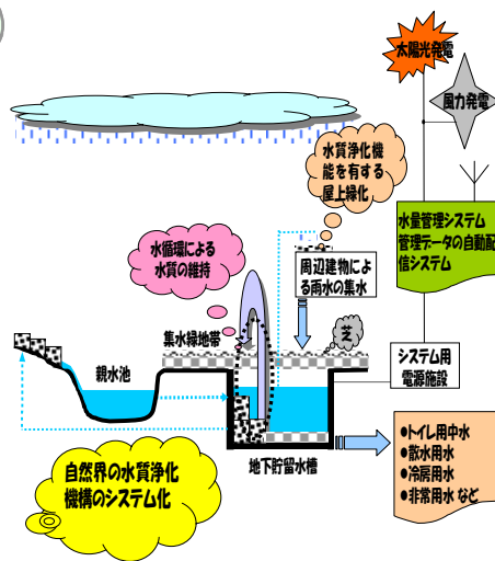
ろ過システムフロー図
