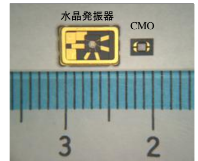
【水晶発振器とCMOのサイズ比較】
