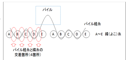
5ピック織り模式図
