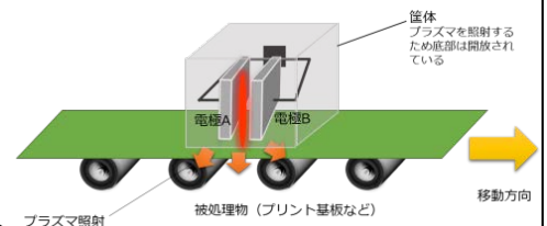
大気圧プラズマ処理装置 イメージ図
