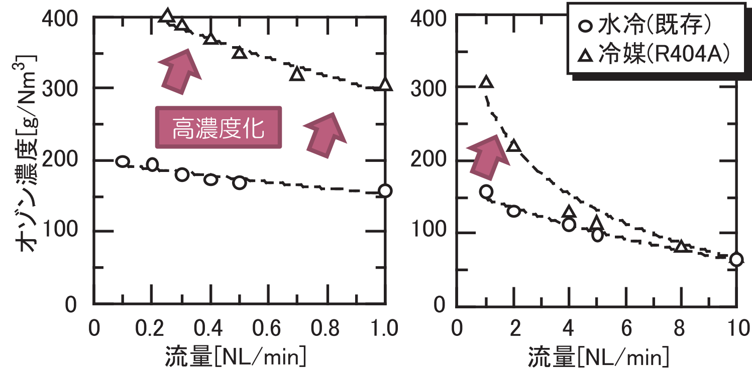
図. 冷却方式によるオゾン濃度の変化
