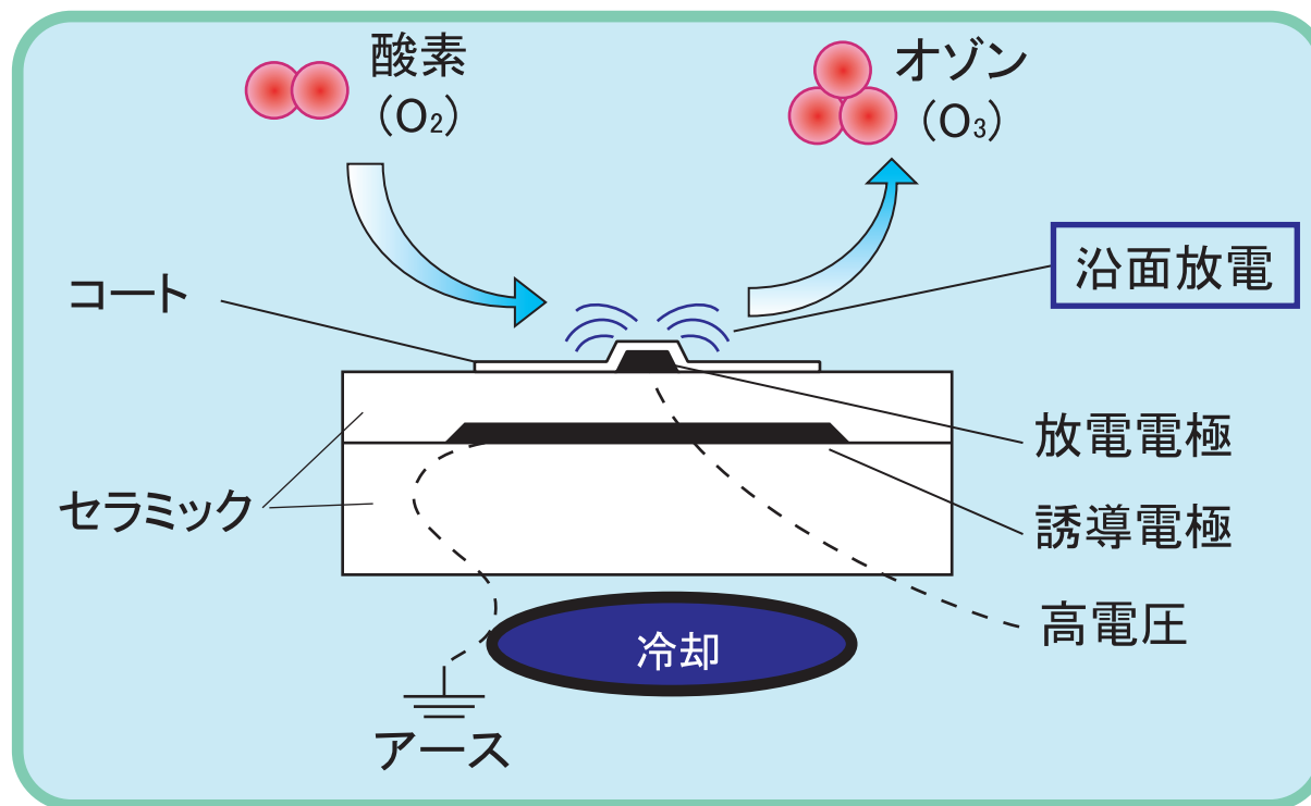
図. 沿面放電の概略
