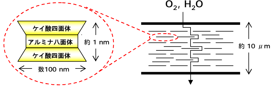
ガスバリア性向上の概念図 (曲路効果)
