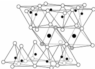
特殊粘土原料(モンモリロナイト)のモデル図
