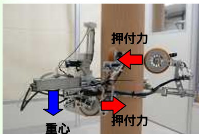
図2 試作機
