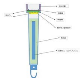
スティックの構造
