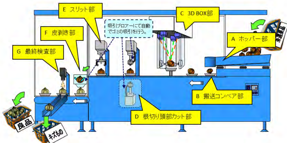
全自動玉葱皮剥き機(イメージ図)
