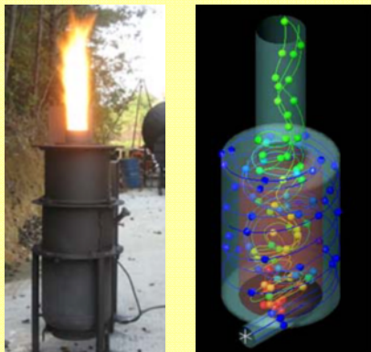
新技術燃焼原理「遠心分離空間分割」 デモ燃焼・炉内の空気の流れと温度域
