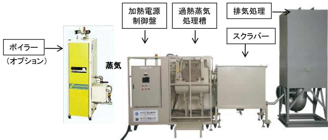
紙おむつ処理装置の外観
