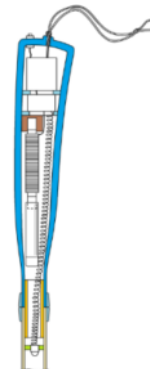
振動発電機内蔵グリップ部
