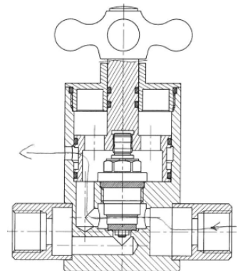
【開発するバルブの構造】
