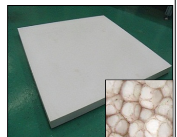
【本事業製品: 防蟻断熱材】
