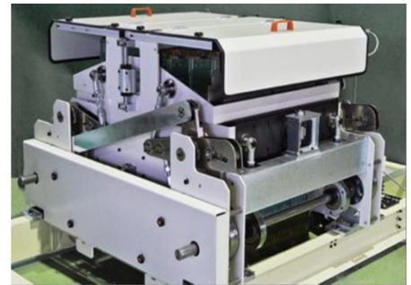
本事業製品 【単動式電子ジャカード】
