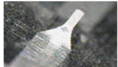
精密角パンチの試作品 □0.020mm (材質:AF1) 刃長:0.15mm / 全長:0.25mm
