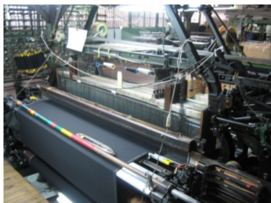
低速織機の「シオンヘル織機」
