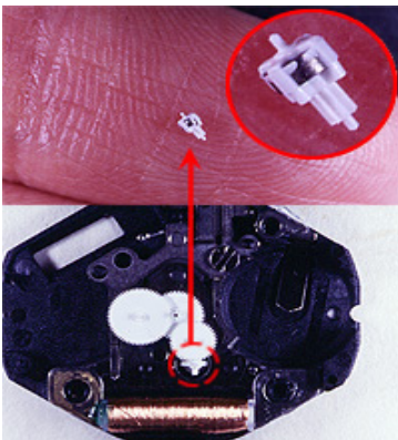
製品名：ローター 用途：腕時計ムーブメント秒針用ギア
