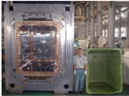
▲ 金型重量215tの射出成型金型
