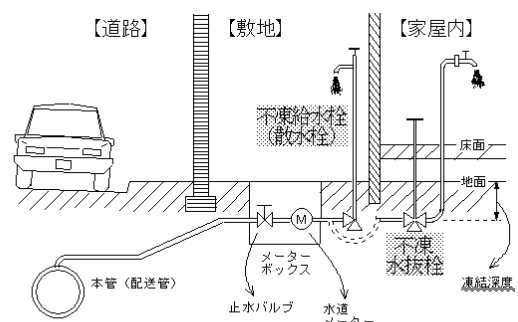
散水栓
