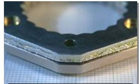
従来のプレスで加工した切口(上) FB加工した平滑な切口(下)
