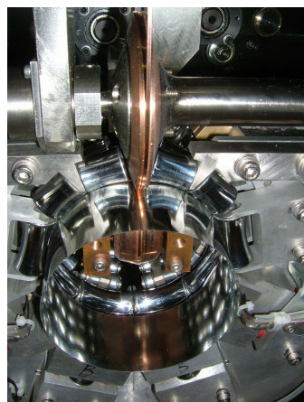
缶製造中(ワイヤーシーム溶接)
